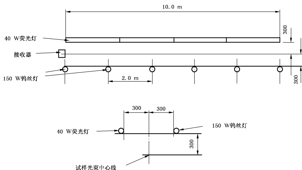
图 1 试验灯布置图
