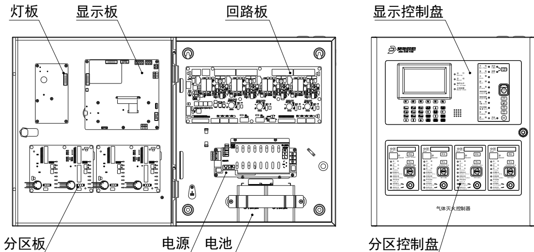
JBF-51S05 结构介绍
