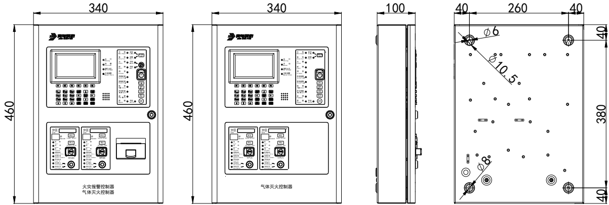
JB-QB-JBF-51S04 / JBF-51S06 尺寸图
