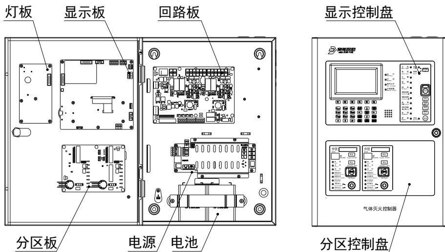
JBF-51S06 结构介绍
