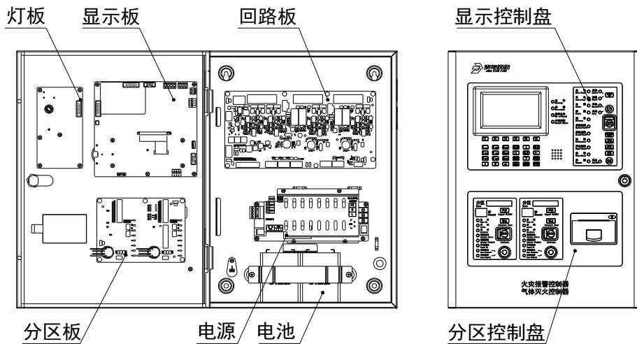
JB-QB-JBF-51S04 结构介绍
