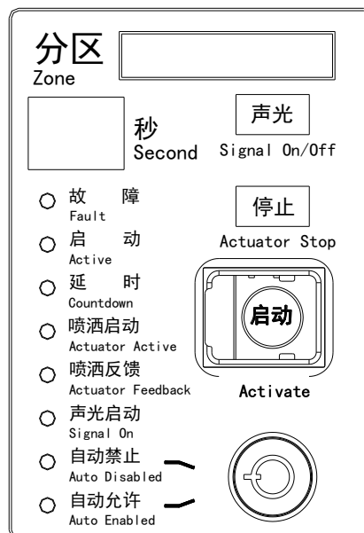
灭火分区面板图
