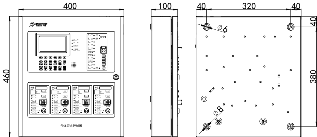
JBF-51S05 尺寸图
