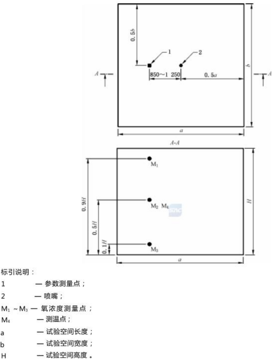
图 13 喷嘴浓度分布试验参数测量点布置示意图
