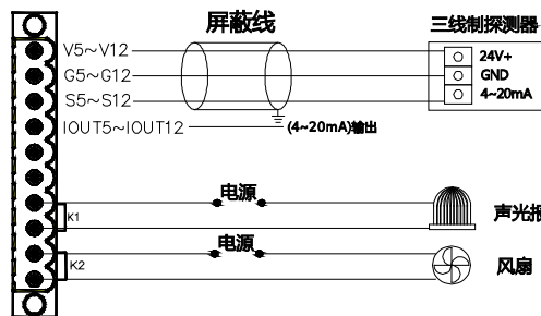
通道卡接线图
