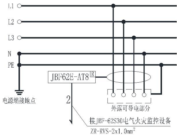
TN-S系统
