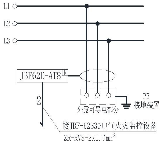
IT系统
