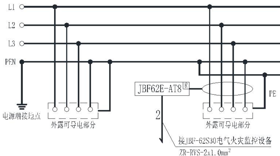
TN-C-S系统
