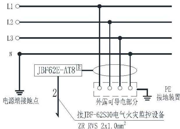
TT系统
