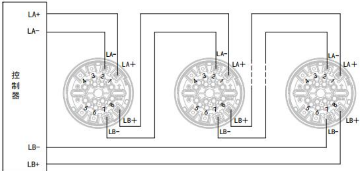
图3 环路接线方式底座接线图
