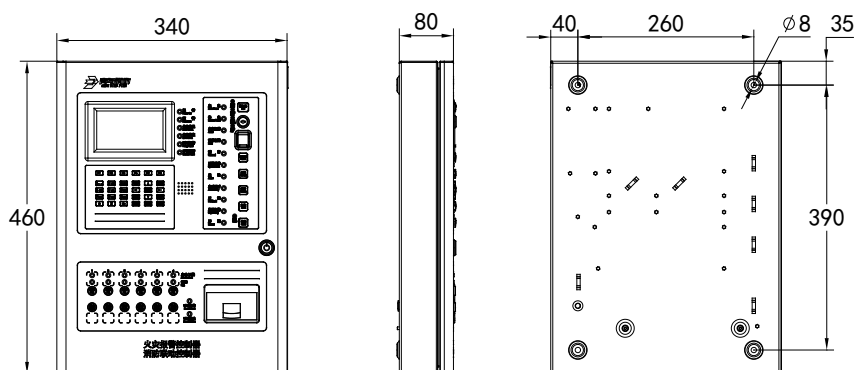
JB-QB-JBF-52S01 尺寸图
