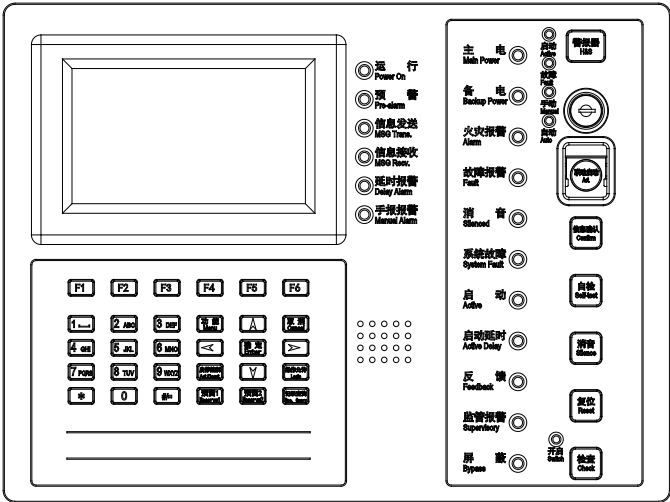
显示盘面板图
