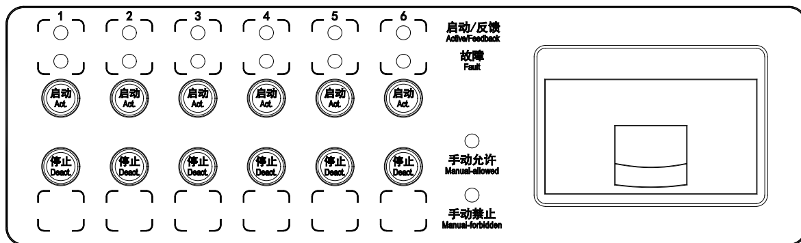
专线盘面板图
