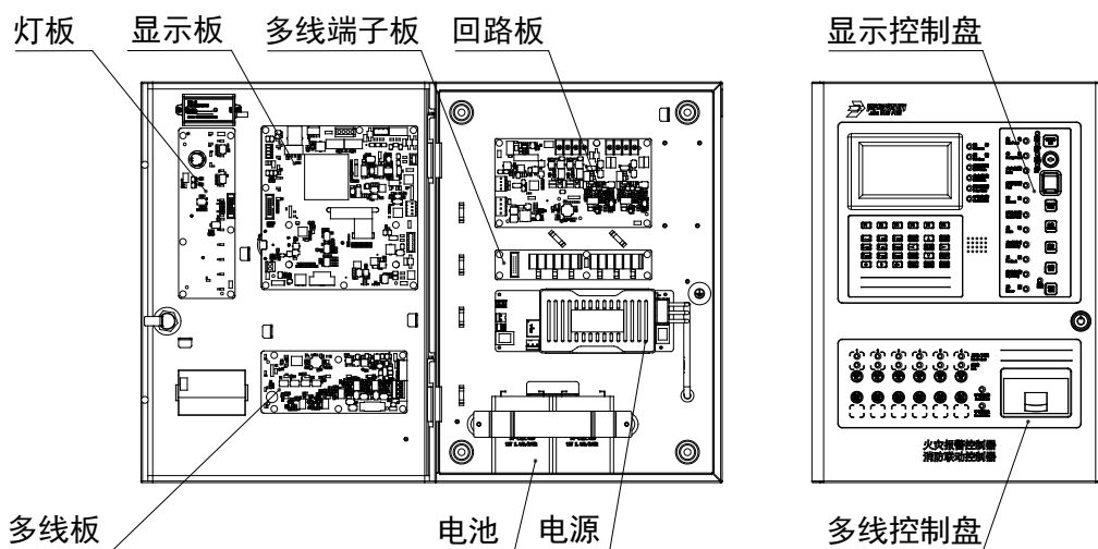
JB-QB-JBF-52S01 结构介绍
