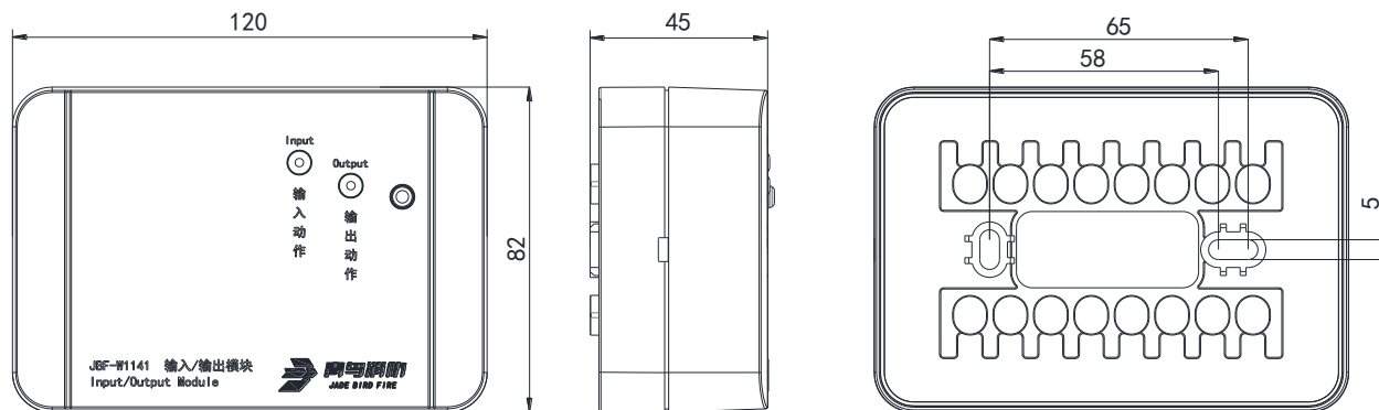
图 1 外形及安装尺寸
