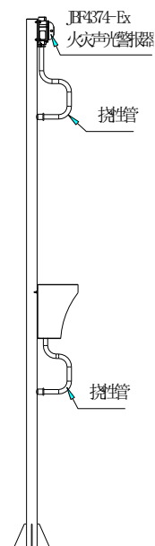
图 6 挠性管走线图
