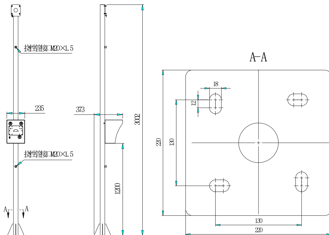
图 2 外形图
