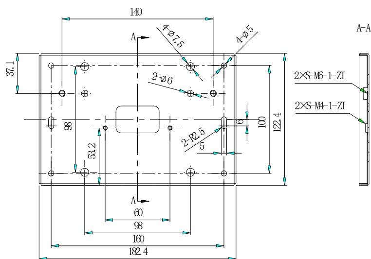
图 5 背板支架安装尺寸图
