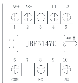
图 2 端子图
