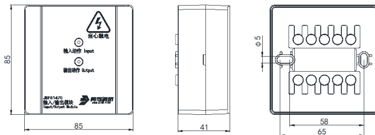
图 1 外形及安装尺寸图
