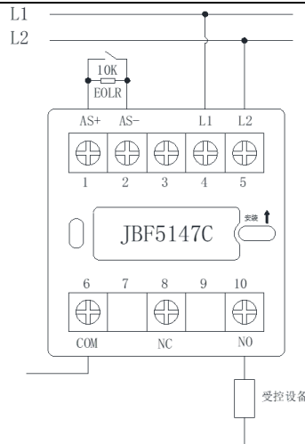
图 3 输出接线方式
