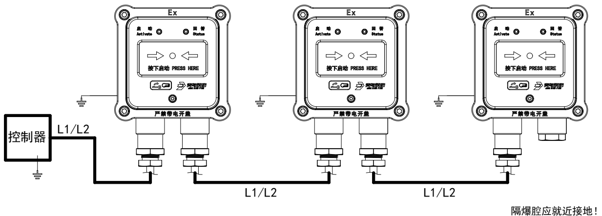
图 2 接线图
