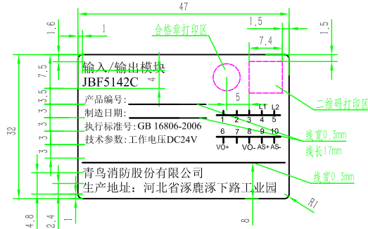
2:1 图样
