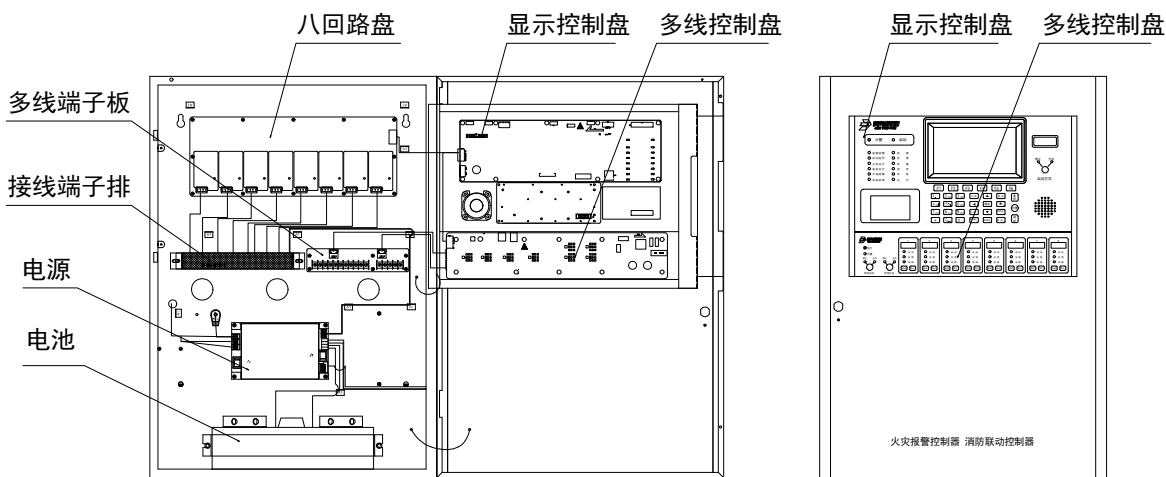
壁挂型控制器结构介绍
