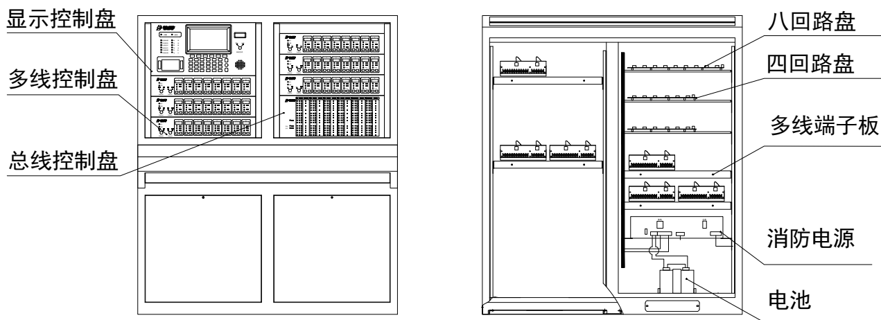
琴台型控制器结构介绍
