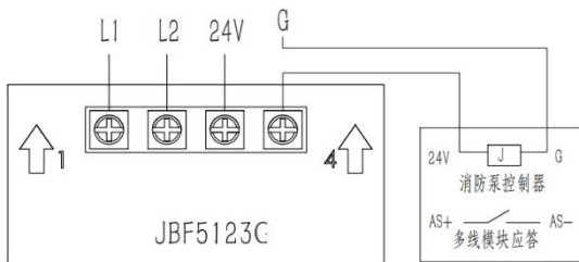
图 2 端子图
