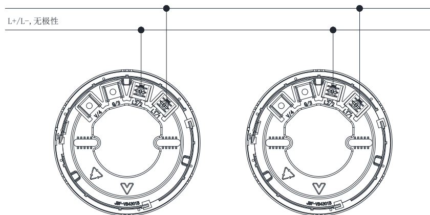
图 2 接线图例
