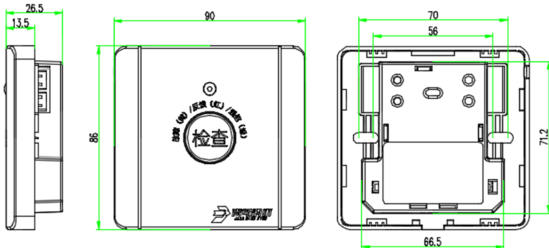
图2 外形及尺寸图（不含底座）
