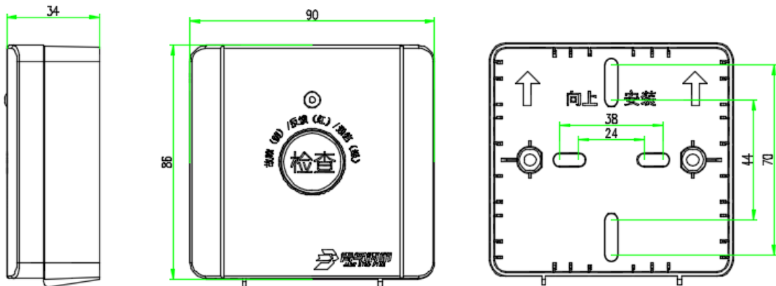
图1 外形及尺寸图（含底座）
