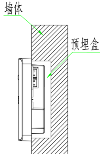
图 3、暗装方式
