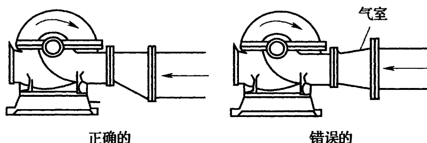
图4 正确和错误的水泵吸水管安装示意
