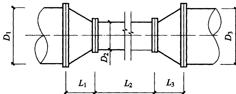
图 3 节流管结构示意
