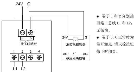
图2 端子接线图
