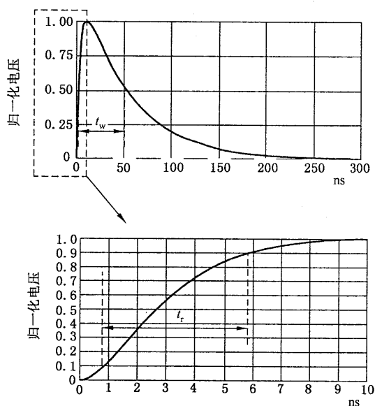
图3 输出到 50 Ω 负载的单个脉冲的理想波形( t_r=5 ns, t_w=50 ns)
