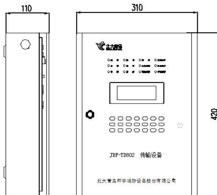
外形尺寸图
