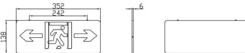
吊装外形尺寸示例
