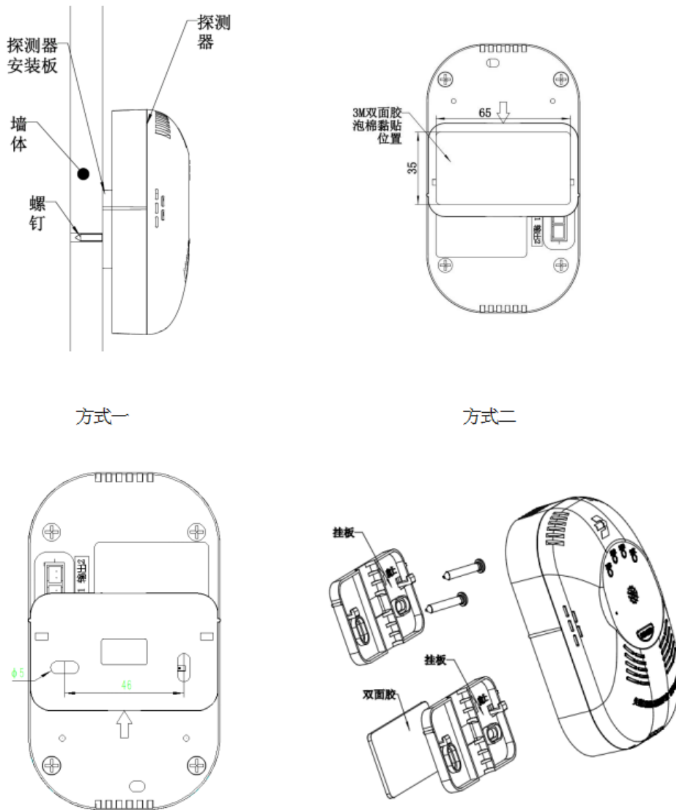
图 1 外形及安装尺寸图
