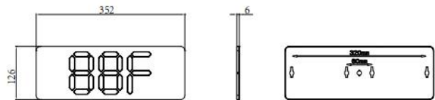
壁挂灯具外形尺寸示意图
