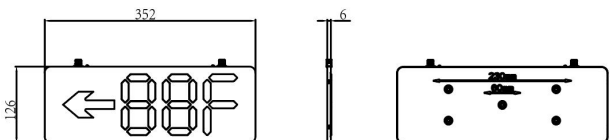
吊装灯具外形尺寸示意图
