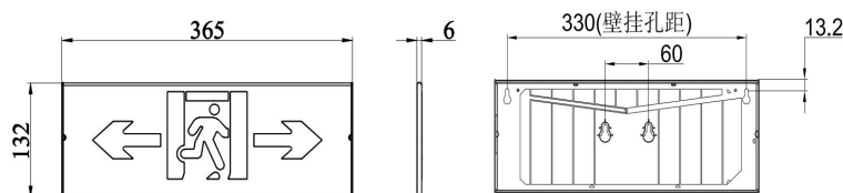
b) 单面壁挂灯具
