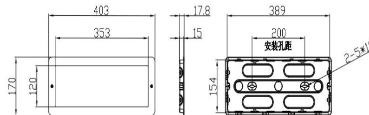
壁挂灯具暗装示意图（J-YMH14 标志灯预埋盒（薄款））
