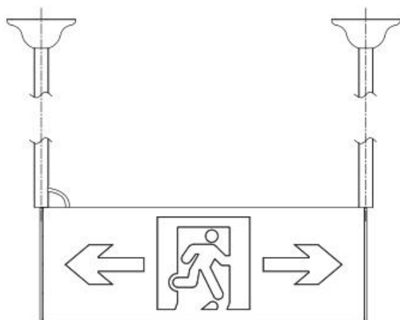
吊装灯具安装示意图
